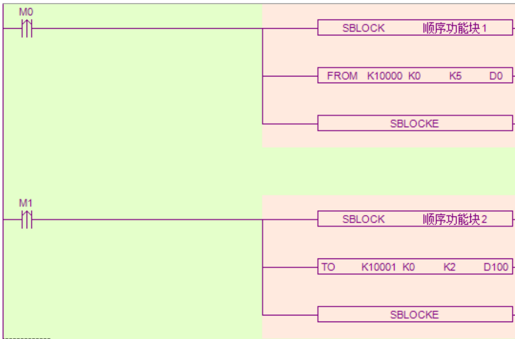
(d) 转化为梯形图
