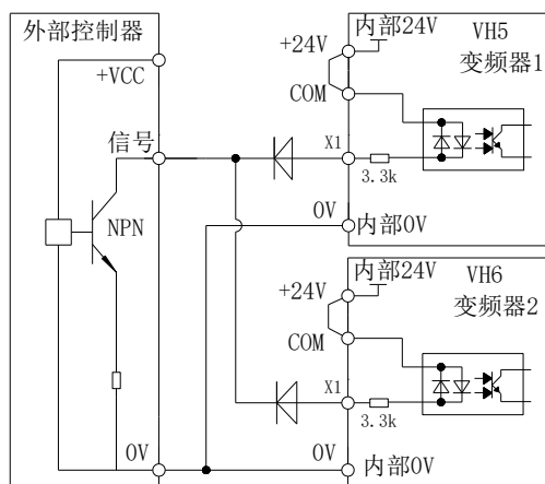
多台变频器使用变频器内部 24V 电源的漏型接线方法
