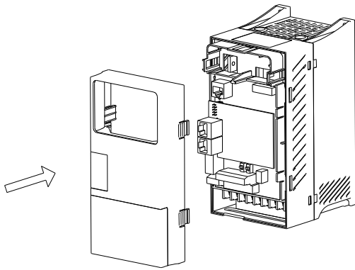
上壳对齐后，沿箭头方向推进去
