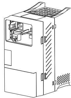
完成上壳安装
